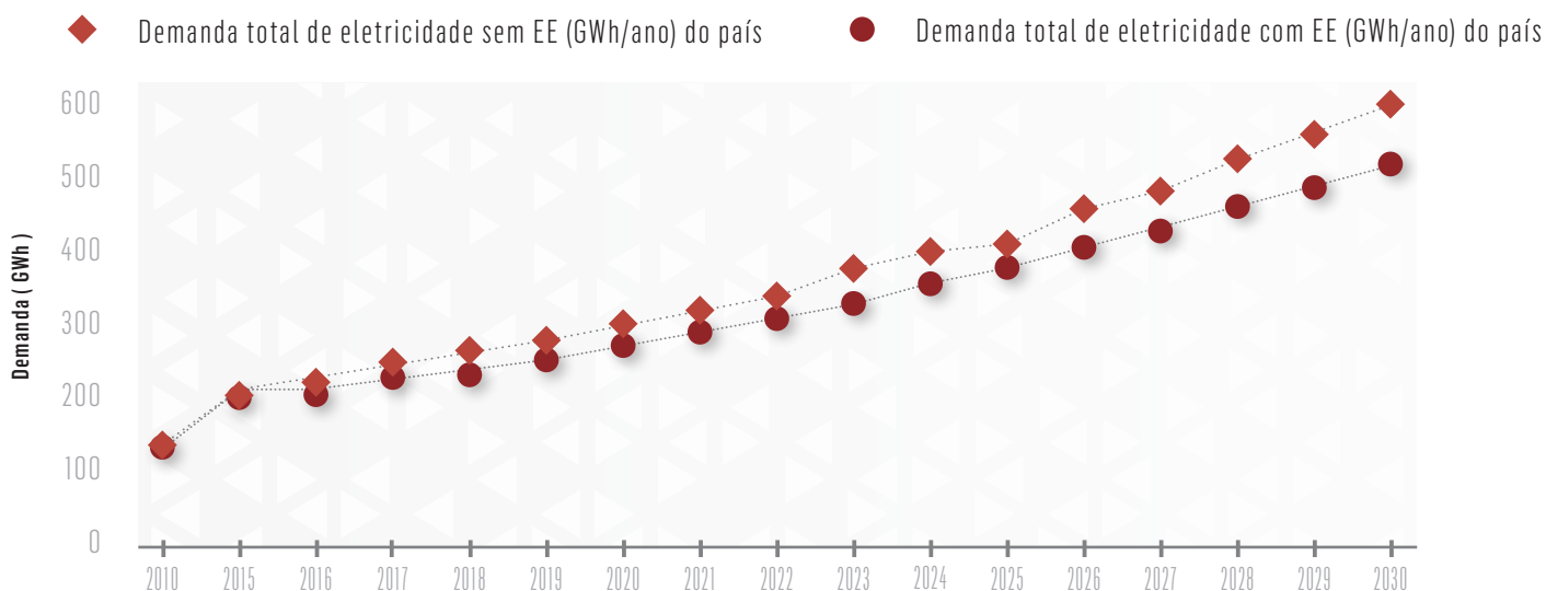
FIGURA 5 Evolução esperada da demanda de eletricidade da rede (GWh/ano) sem e com medidas de eficiência energética
