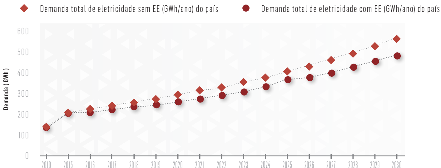
FIGURA 4 Evolução esperada da demanda total de eletricidade (GWh/ano) sem e com medidas de eficiência energética
