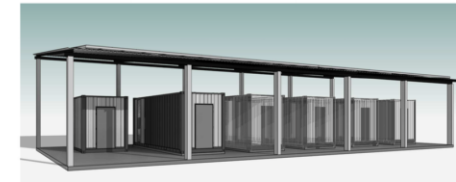
SISTEMA DE CONSERVAÇÃO DE VARIOS PRODUCTOS AGRICOLA E SALA DE CONTROLE ENERGETICAMENTE AUTOSUFICIENTE (DIFERENTES TEMPERATURA)
