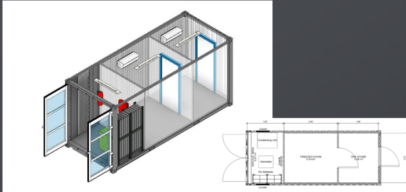
CONTENTOR COM CAMARA PARA PROCESSAMENTO DE PEIXE E CÂMERA FRIA ENERGETICAMENTE AUTOSUFICIENTE
