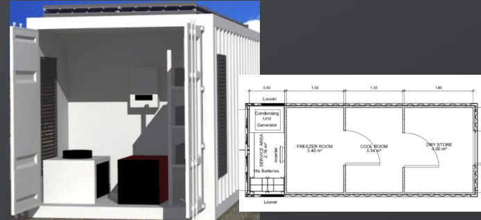
CONTENTOR COM SISTEMA FV PARA CÂMERAS FRIAS (DIFERENTES TEMPERATURA) ENERGETICAMENTE AUTOSUFICIENTE
